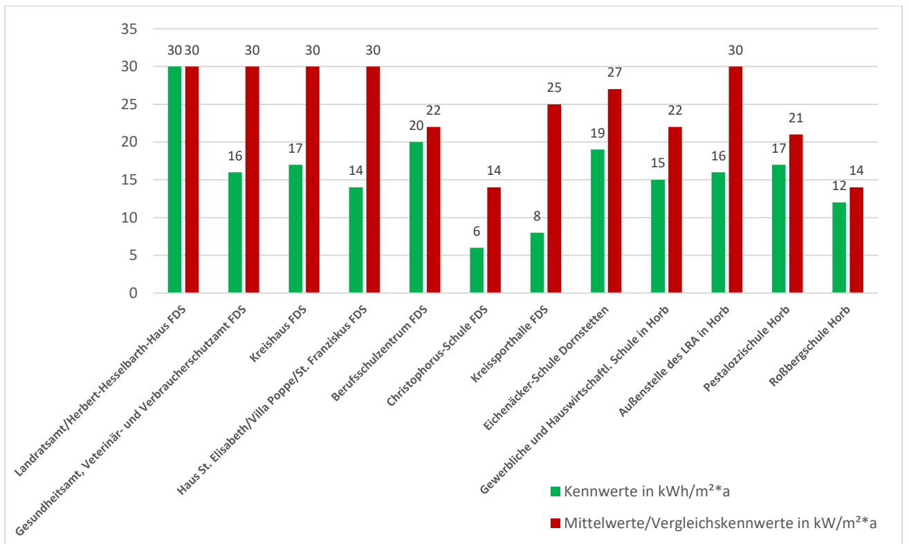
Abbildung 8: Stromenergieverbrauch: Kenn- und Vergleichswerte
