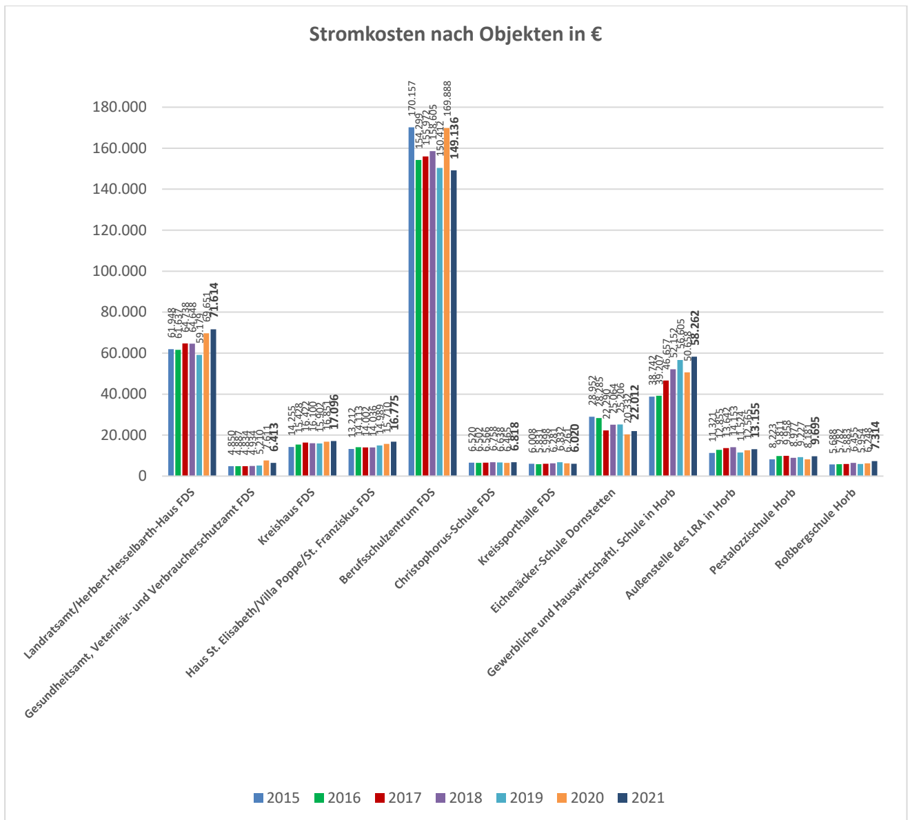
Abbildung 12: Stromenergieverbrauch, jährliche Kosten in €
