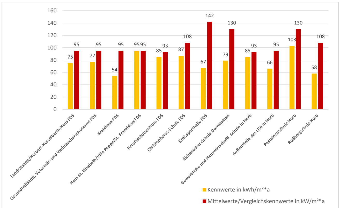
Abbildung 7: Heizenergieverbrauch (witterungsbereinigt): Kenn- und Vergleichswerte
