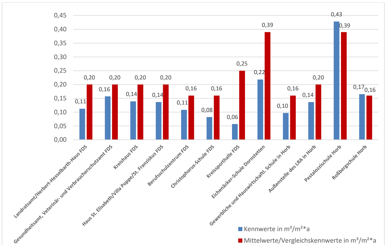
Abbildung 9: Wasserverbrauch: Kenn- und Vergleichswerte
