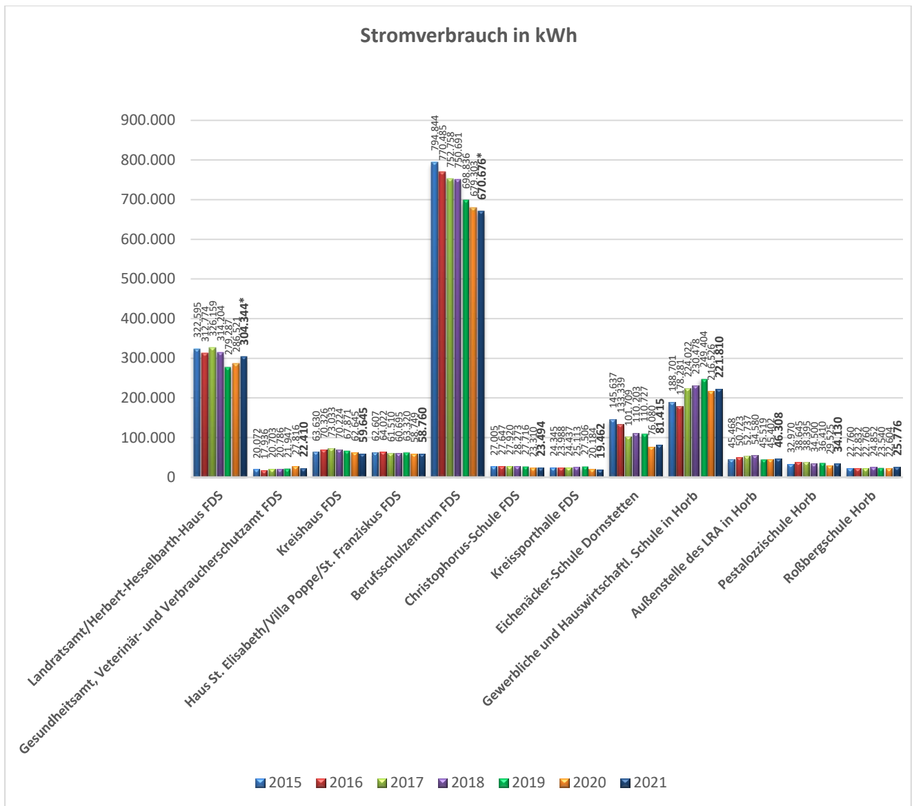
Abbildung 5: Stromenergieverbrauch
