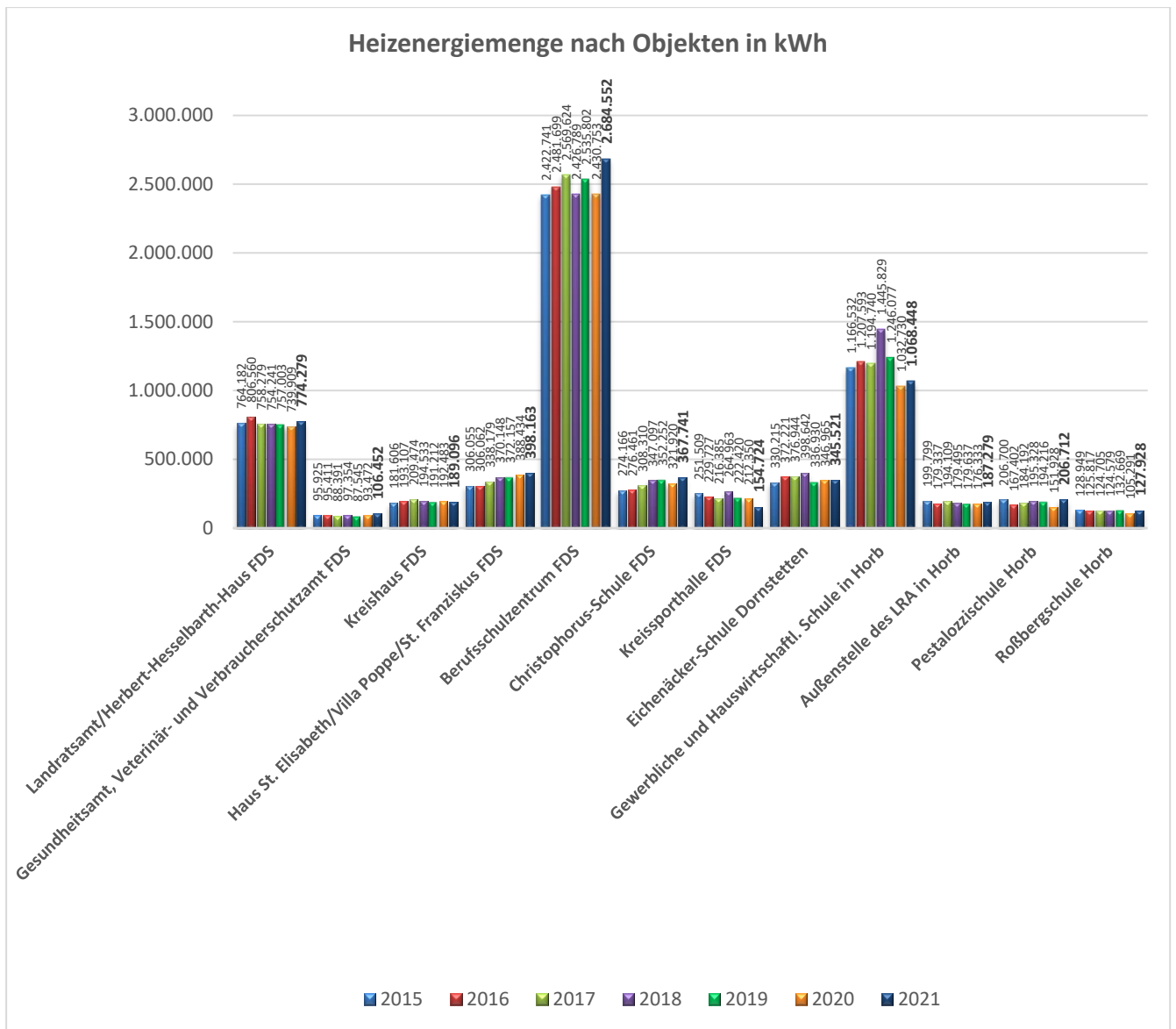
Abbildung 4: Heizenergieverbrauch (witterungsbereinigt)
