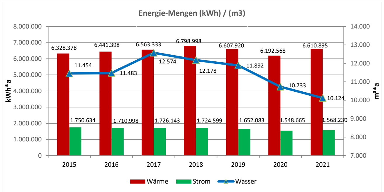
Abbildung 2: Energiemengen (Heizenergie-witterungsbereinigt) gesamt für 12 Liegenschaften
